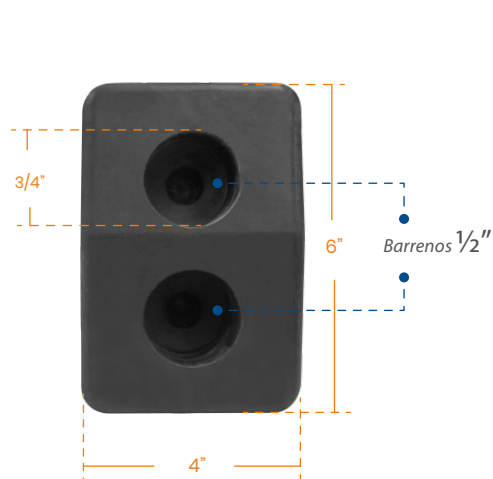
ANCHO Y ALTO DEL TOPE Vista frontal.
